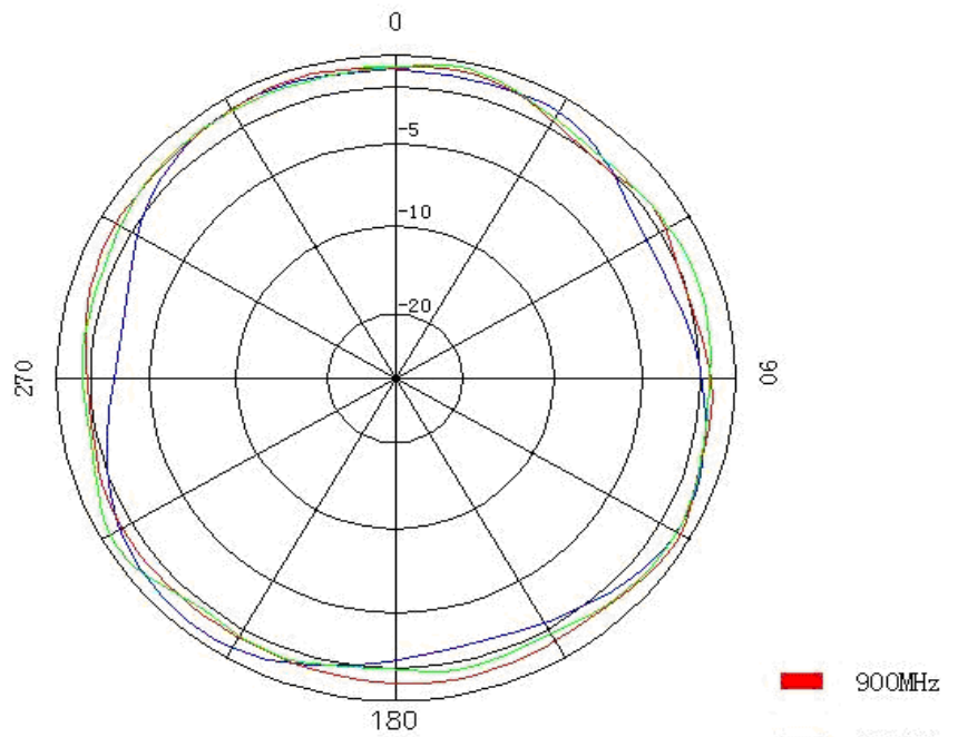
水平面方向图 Horizontal Pattern
