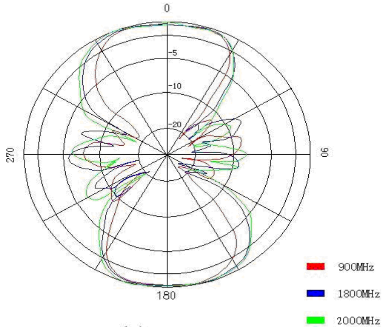
垂直面方向图 Vertical Pattern
